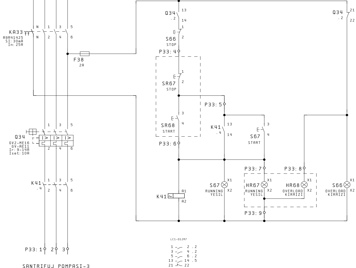
SANTRIFUJ POMPASI-3 5.5kW
