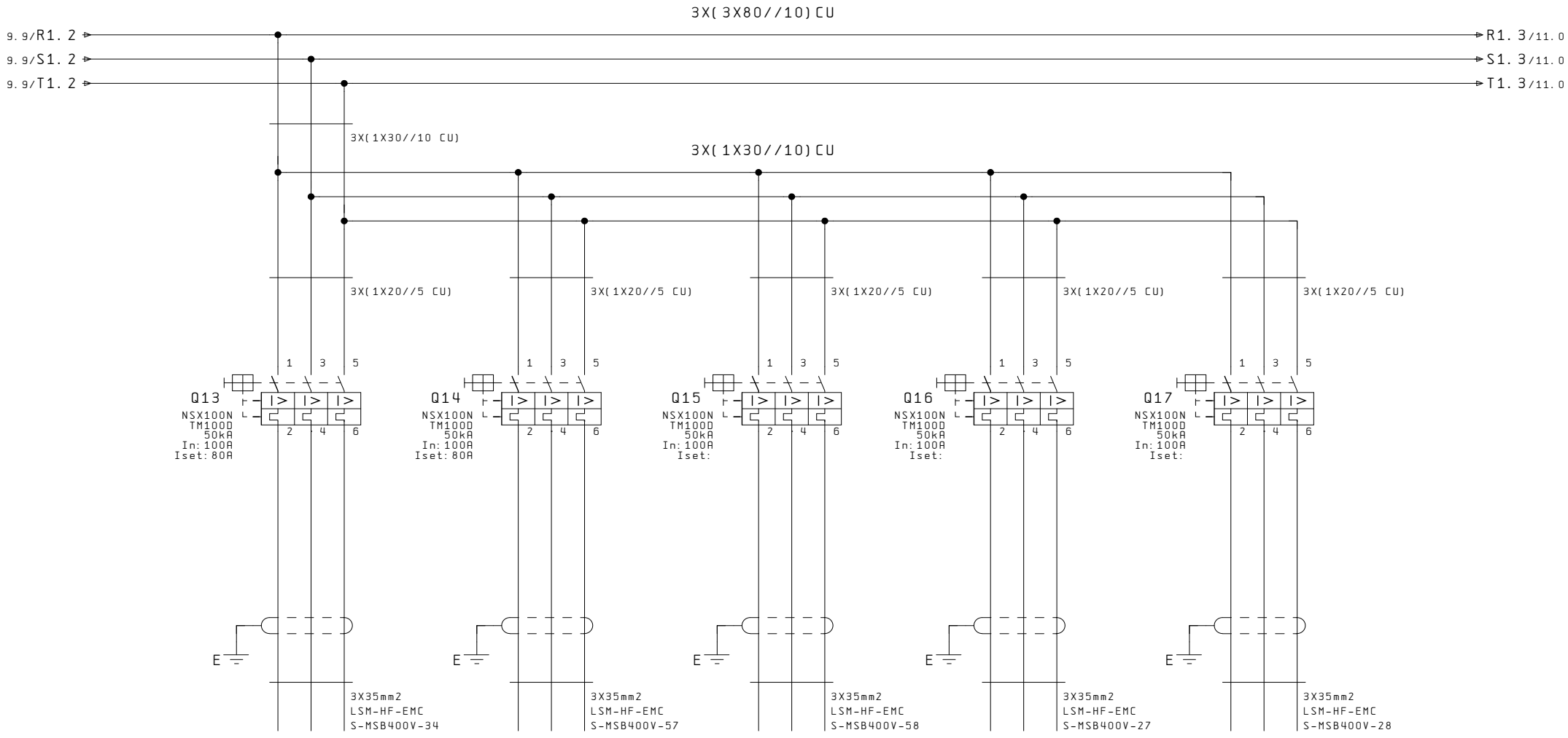
NO. 5 HAVUZ BORDA PRIZ PANOSU
