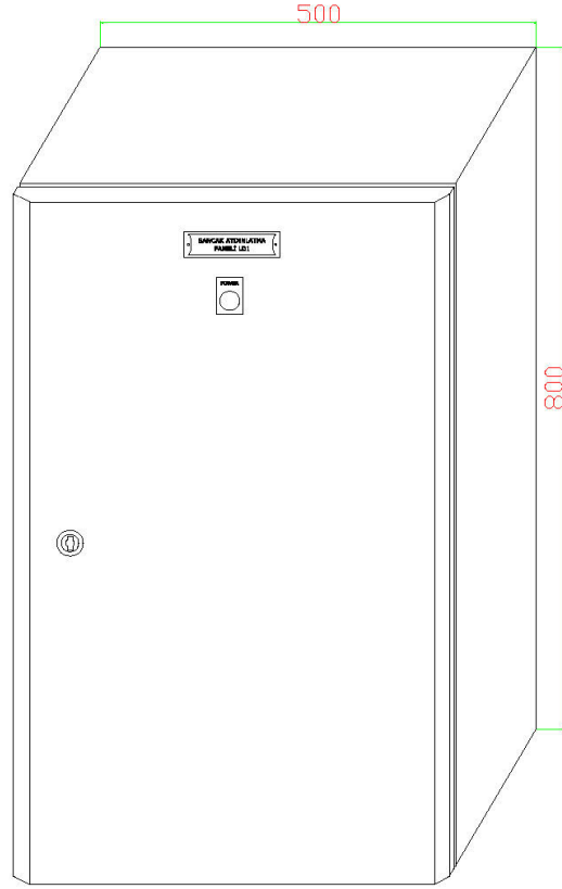
ÖNDEN GÖRÜNÜŞ
