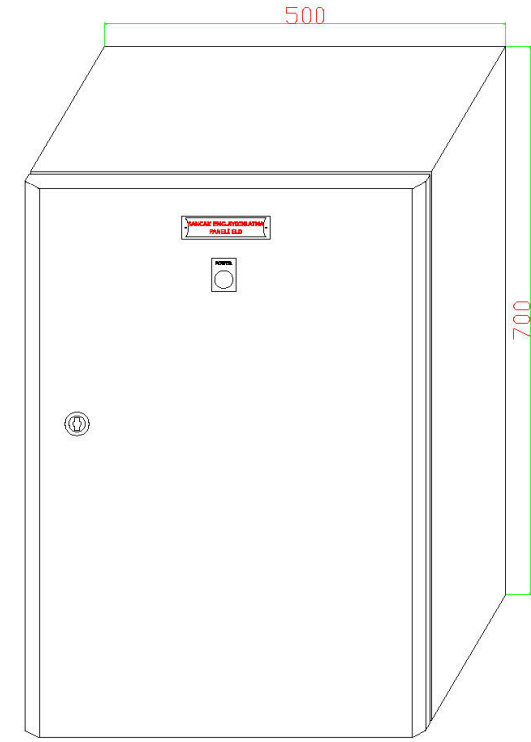
ÖNDEN GÖRÜNÜŞ
